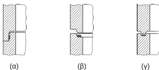
Σχήμα 4 - Τυπικές συνδέσεις σπονδύλων
