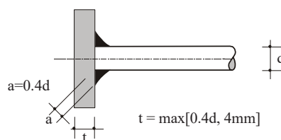
Σχήμα 14 - Μετωπική συγκόλληση ράβδου
