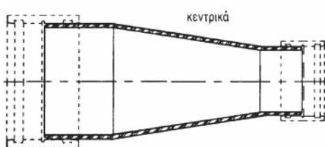
Σχήμα 8 - Συμμετρικό συστολικό
