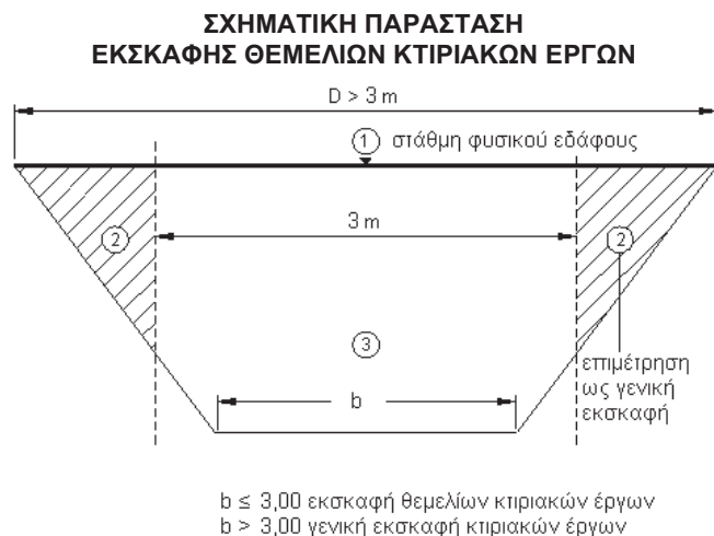
Σχήμα 1: Επιμέτρηση εκσκαφών κτιριακών έργων
