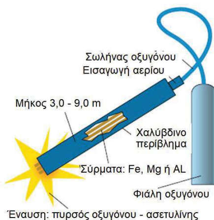
Εικόνα 1 Λειτουργικό διάγραμμα θερμικής λόγχης
