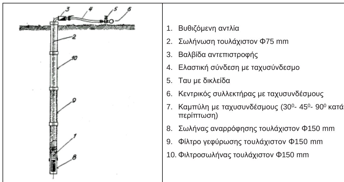
Σχήμα 1 - Σχηματική παράσταση βαθέος διασωληνωμένου φρέατος
