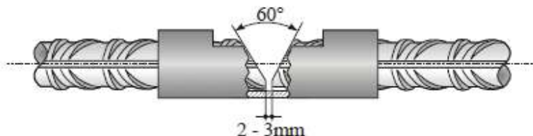
Σχήμα 7 Μετωπική σύνδεση με υποστήριξη της ρίζας της συγκόλλησης [πηγή: KTX 2008]
