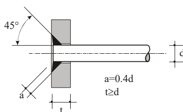
Σχήμα 14 - Ράβδος χωνευτή στο έλασμα
