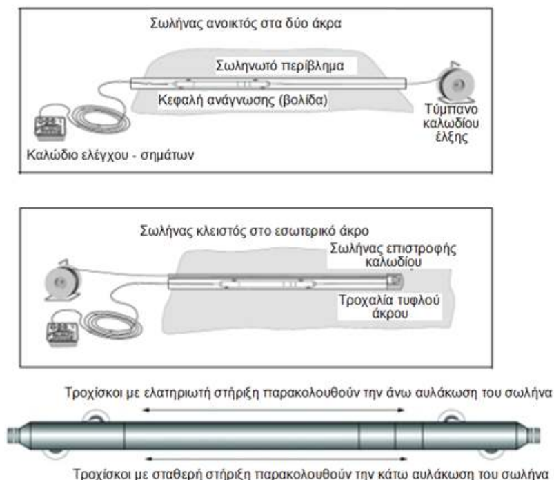
Σχήμα 1 - Διάταξη οριζόντιου κλισιομέτρου (Πηγή: Βιβλιογραφία [5])
