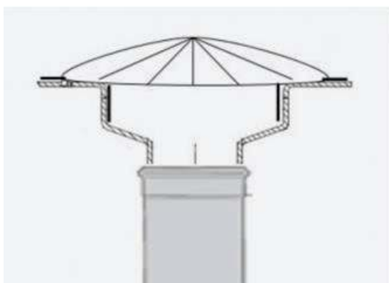
Εικόνα 1 - Ενδεικτικές διαμορφώσεις κυκλικών φρεατίων υδροσυλλογής καταστρώματος γεφυρών κατά ΕΛΟΤ EN 124-1
