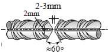
Σχήμα 8 - Εναλλακτική προετοιμασία οπλισμών [πηγή: KTX 2008 8.4.2 Σχ.(α)]
