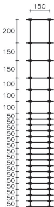
Σχήμα 1. Βασικά χαρακτηριστικά συρματοπλέγματος τύπου URSUS 160/23/15
