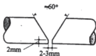
Σχήμα 5 Λοξοτομή μονού-V στις δύο ράβδους σε οριζόντια θέση [πηγή: KTX 2008]
