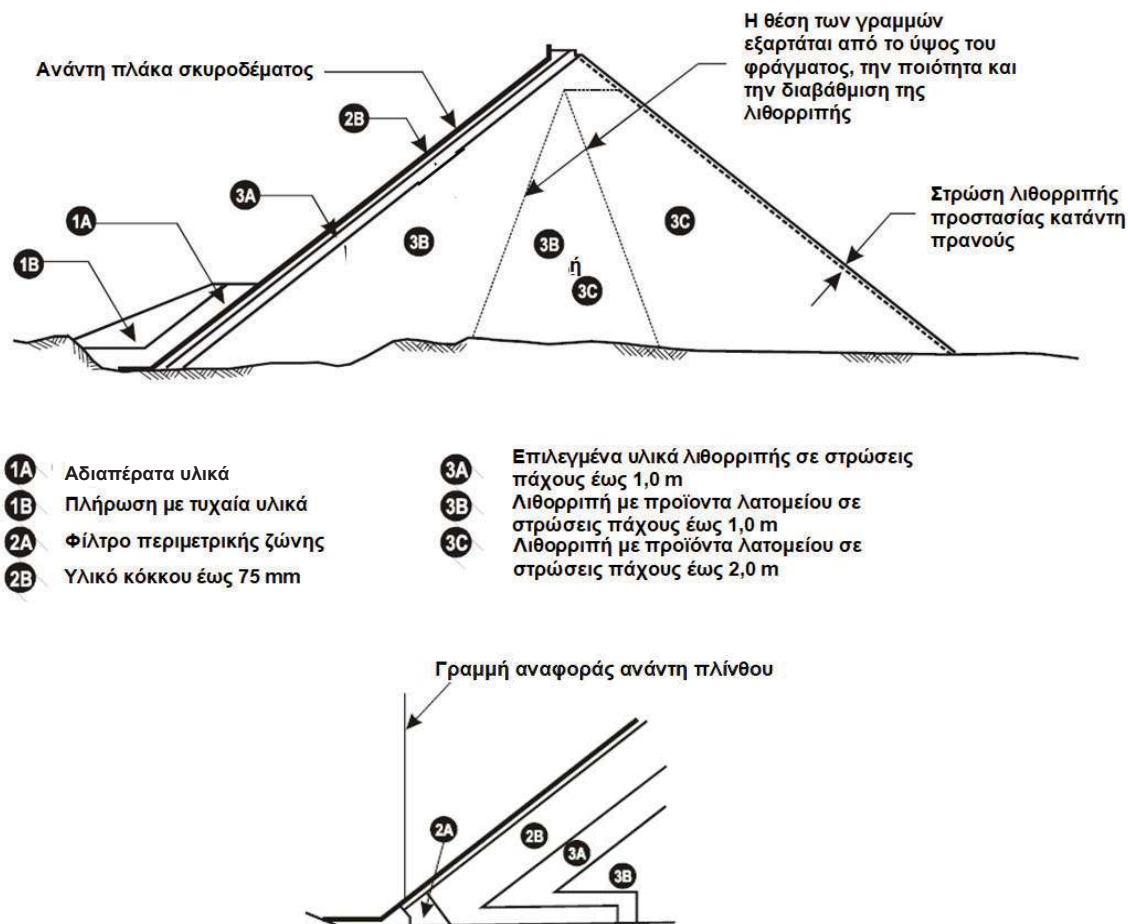
Σχήμα 1 - Τυπική διαζώνιση λιθορριπτού φράγματος με ανάτη πλάκα σκυροδέματος
