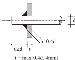
Σχήμα 13 - Ράβδος διερχόμενη από το έλασμα
