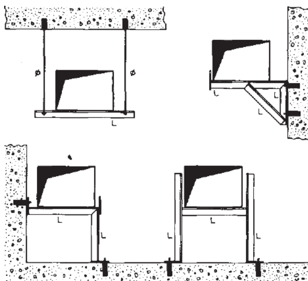
Σχήμα 7 - Στήριξεις/αναρτήσεις αεραγωγών
