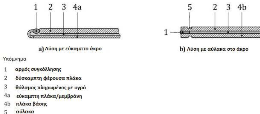
Σχήμα 3 Παραδείγματα τεχνικών λύσεων για την ελαχιστοποίηση της συγκέντρωσης τάσεων στις άκρες
