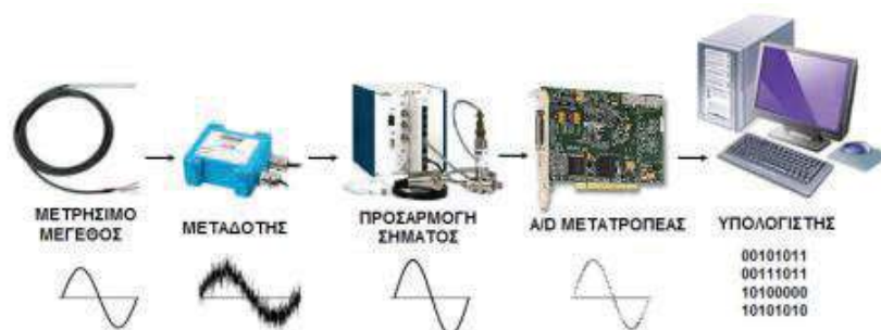
Εικόνα 2 - Διαδικασία επεξεργασίας σημάτων αισθητήρων
