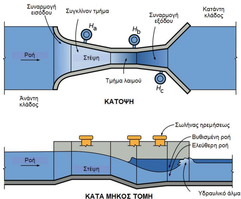
Σχήμα 1 - Διάταξη Parshall
