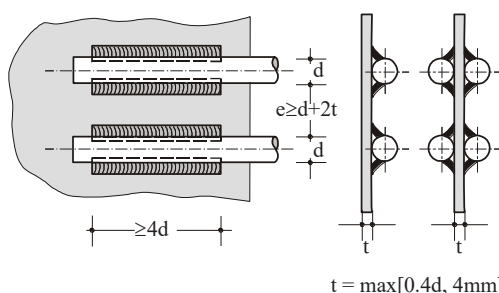
Σχήμα 12 - Αμφίπλευρη συγκόλληση [πηγή: ΚΤΧ 2008]
