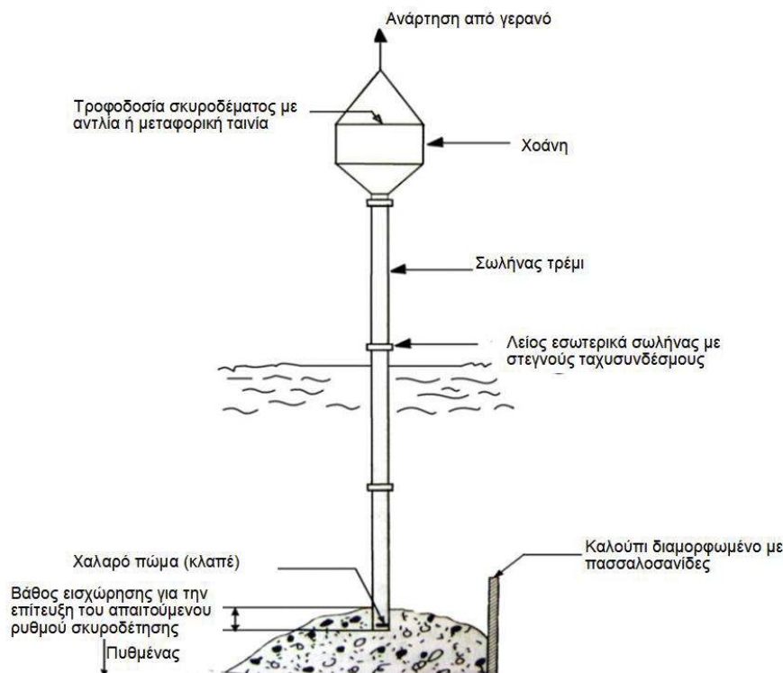
Σχήμα 1 - Ύψαλη σκυροδέτηση με καθοδηγητικό σωλήνα (tremie pipe)
