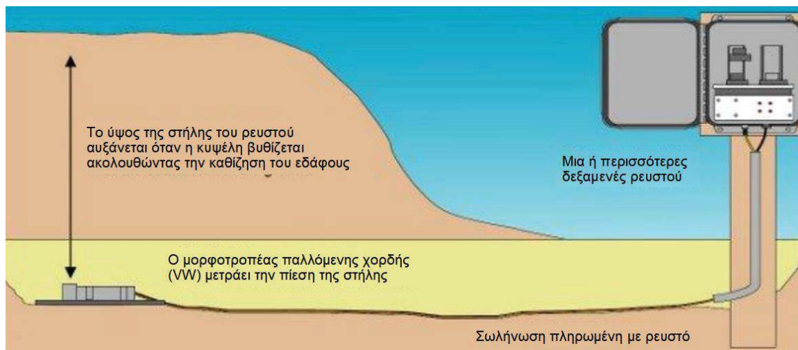
Σχήμα 1 - Γενική διάταξη και λειτουργία υδραυλικού καθιζισιμέτρου
