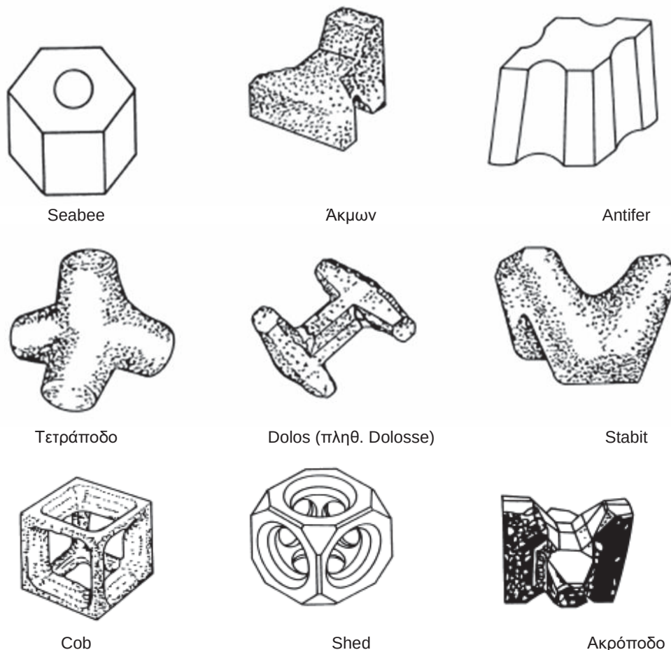
Σχήμα 1 - Μερικοί από τους συνηθέστερους τύπους Ειδικών Τεχνητών Ογκολίθων
