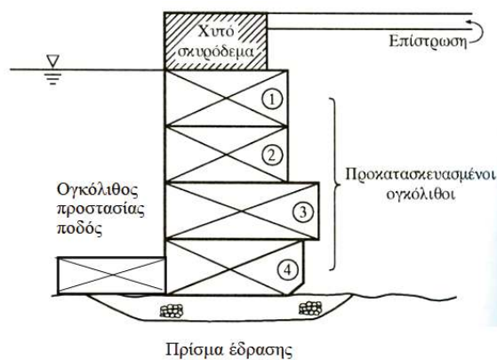
Σχήμα 1 - Παράδειγμα διατομής κρηπιδοτοιχίου
