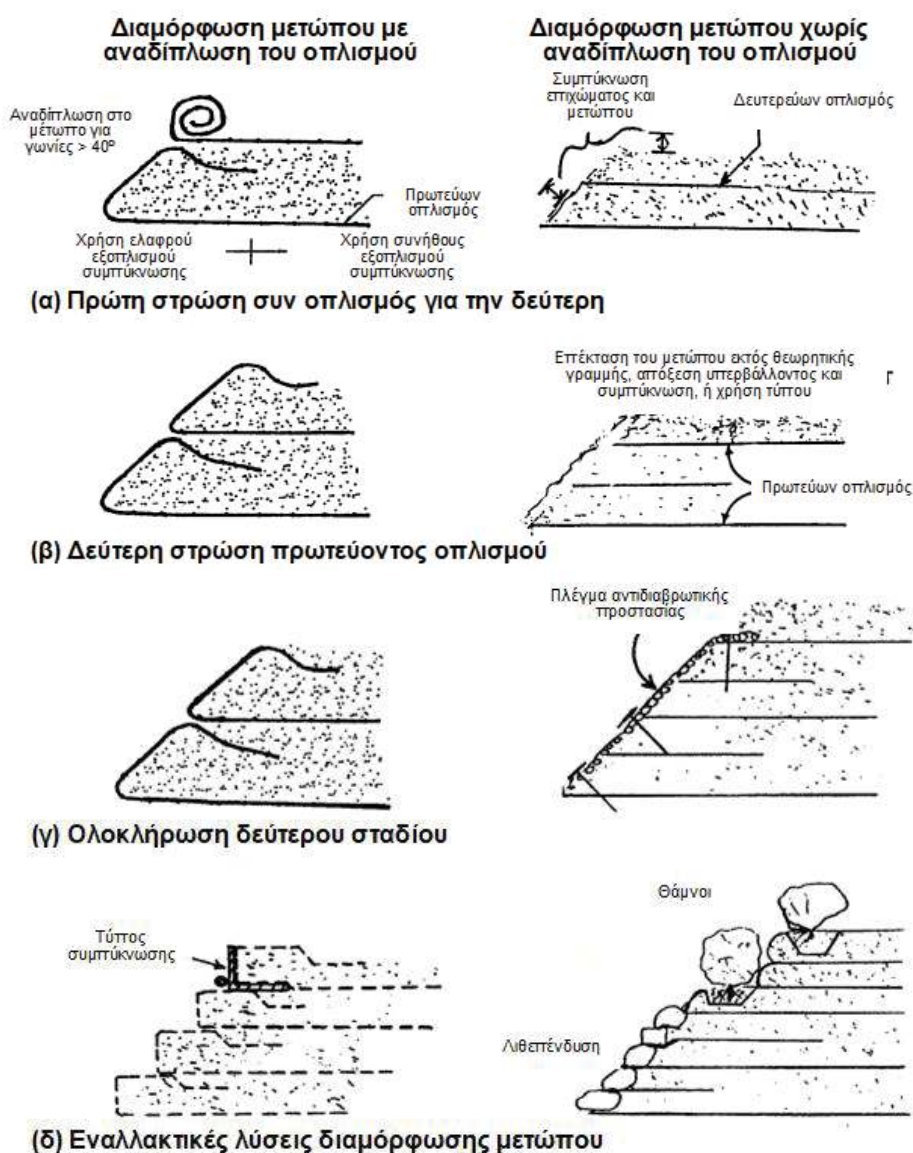
Σχήμα 2 - Επένδυση πρανού οπλισμένου επιχώματος με αναδιπλούμενα και αγκυρούμενα γεωσυνθετικά
