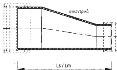
Σχήμα 9 - Έκκεντρο συστολικό
