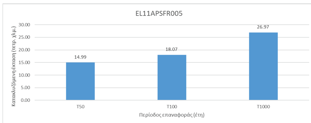
Σχήμα 3-9: Κατακλυζόμενες εκτάσεις ΖΔΥΚΠ EL11APSFR005 για τις πλημμύρες περιόδου επαναφοράς 50, 100 και 1.000 ετών
