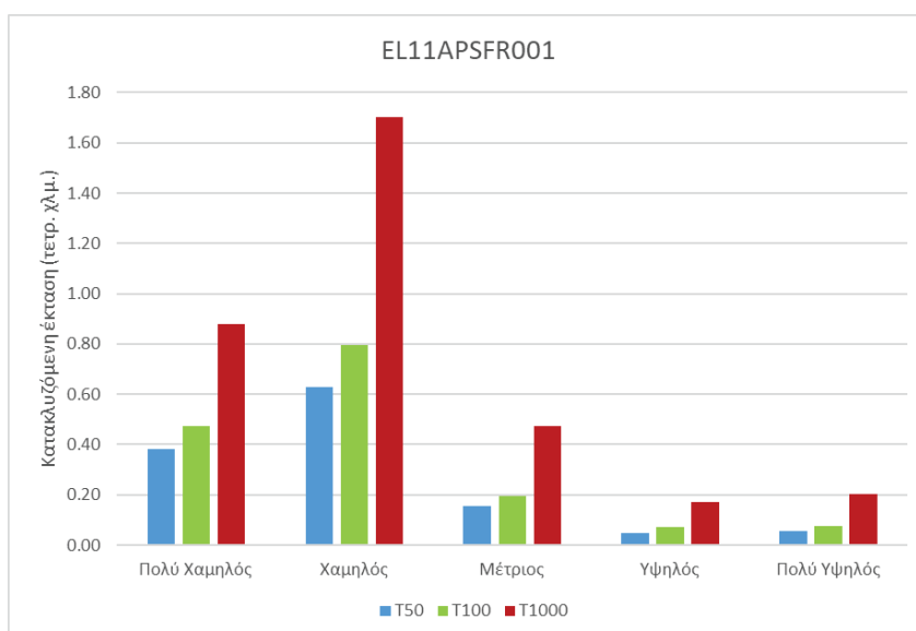
Σχήμα 3-14: Κατακλυζόμενη έκταση που αντιστοιχεί σε κάθε κατηγορία του δείκτη Επικινδυνότητας Πλημμύρας (κλάση Βαθμού Επιρροής Πλημμύρας), ανά εξεταζόμενο σενάριο στο σύνολο της ΖΔΥΚΠ EL11APSF001
