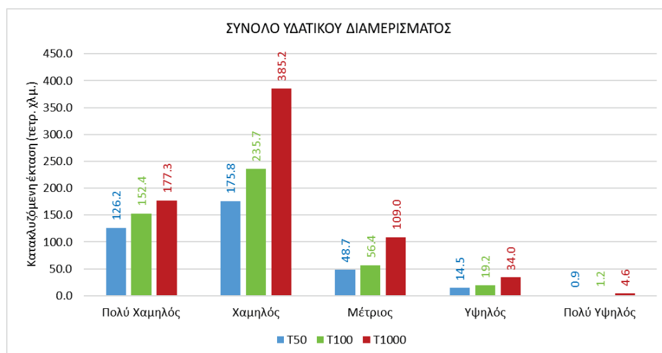
Σχήμα 4-2: Κατακλυζόμενες εκτάσεις ανά κλάση Κινδύνου Πλημμύρας (κλάση Επιπτώσεων Πλημμύρας) και ανά εξεταζόμενο σενάριο (σύνολο ΥΔ EL11)
