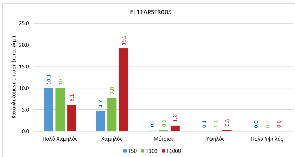
Εικόνα 4-5: Έκταση που αντιστοιχεί σε κάθε κατηγορία κινδύνου πλημμύρας, ανά περίοδο επαναφοράς (ΖΔΥΚΠ EL11APSF005)
