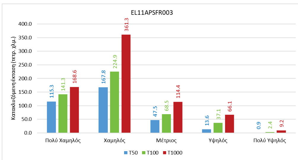
Εικόνα 4-3: Έκταση που αντιστοιχεί σε κάθε κατηγορία κινδύνου πλημμύρας, ανά περίοδο επαναφοράς (ΖΔΥΚΠ EL11APSFR003)
