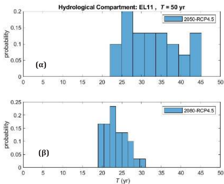
Σχήμα 3-29: Ποσοστά των σταθμών του ΥΔ11 ως συνάρτηση των νέων περιόδων επαναφοράς γεγονότων βροχής που, κατά την τρέχουσα περίοδο, αντιστοιχούν σε περίοδο επαναφοράς T = 50 έτη: α) μελλοντική περίοδος 2041-01-01 έως 2070-12-31 (2050s), και β) μελλοντική περίοδος 2071-01-01 έως 2100-12-31 (2080s).
