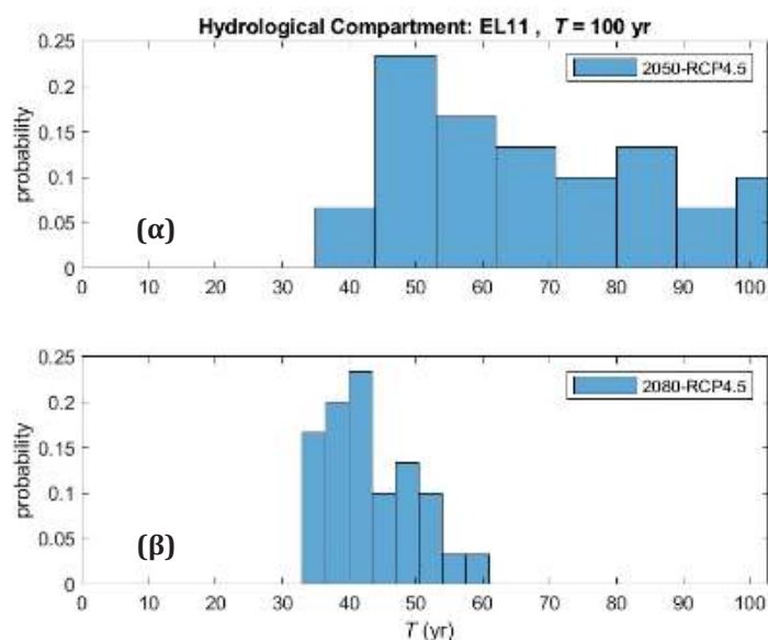
Σχήμα 3-30: Ποσοστά των σταθμών του ΥΔ11 ως συνάρτηση των νέων περιόδων επαναφοράς γεγονότων βροχής που, κατά την τρέχουσα περίοδο, αντιστοιχούν σε περίοδο επαναφοράς T = 100 έτη: α) μελλοντική περίοδος 2041-01-01 έως 2070-12-31 (2050s), και β) μελλοντική περίοδος 2071-01-01 έως 2100-12-31 (2080s).
