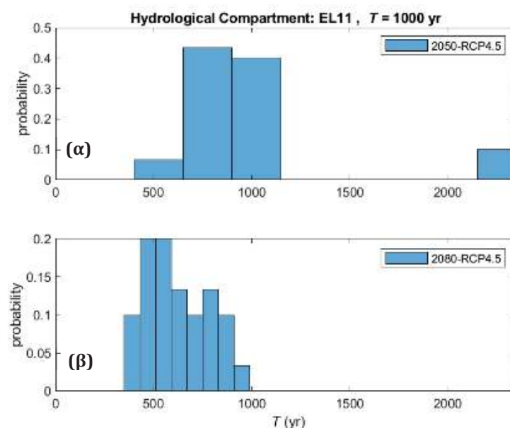
Σχήμα 3-31: Ποσοστά των σταθμών του ΥΔ11 ως συνάρτηση των νέων περιόδων επαναφοράς γεγονότων βροχής που, κατά την τρέχουσα περίοδο, αντιστοιχούν σε περίοδο επαναφοράς T = 1000 έτη: α) μελλοντική περίοδος 2041-01-01 έως 2070-12-31 (2050s), και β) μελλοντική περίοδος 2071-01-01 έως 2100-12-31 (2080s).
