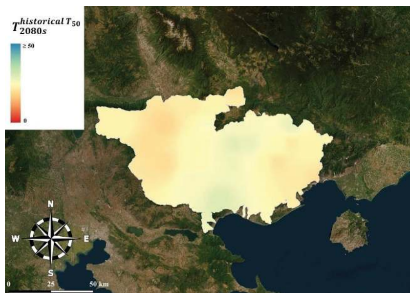
Εικόνα 3-51: Θεματικός χάρτης της χωρικής κατανομής των νέων περιόδων επαναφοράς T_{2080s}^{historical T_x} , για την κλιματική περίοδο 2071-01-01 έως 2100-12-31 (2080s), των γεγονότων βροχής που κατά την τρέχουσα περίοδο αντιστοιχούν σε περιόδους επαναφοράς T = 50 έτη.
