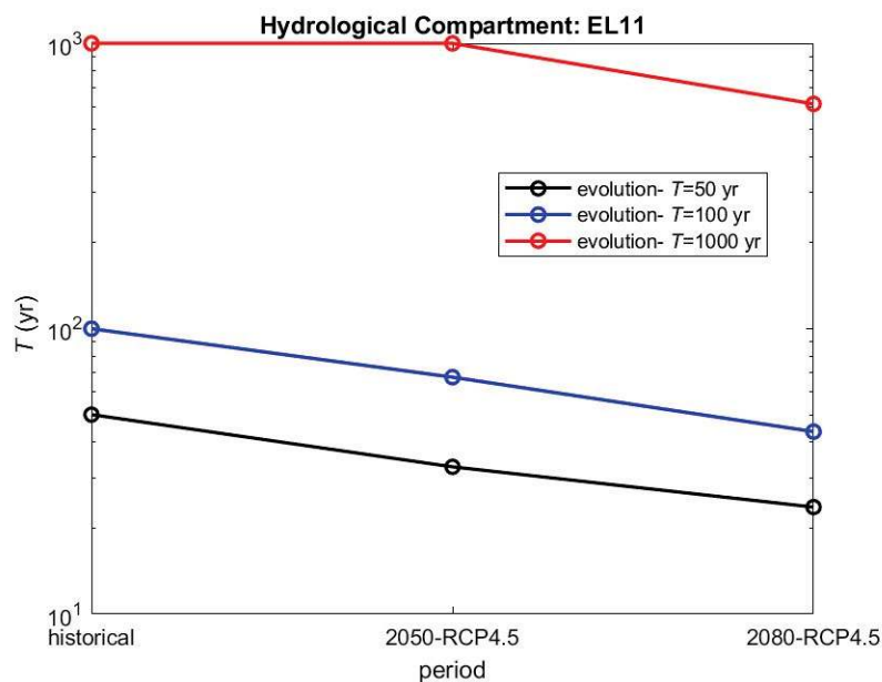
Σχήμα 3-28: Μεταβολή της μέσης περιόδου επαναφοράς στο ΥΔ EL11 κατά τις μελλοντικές περιόδους 2041-01-01 έως 2070-12-31 (2050s) και 2071-01-01 έως 2100-12-31 (2080s).
