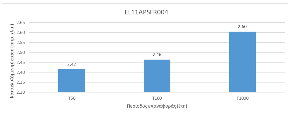
Σχήμα 3-8: Κατακλυζόμενες εκτάσεις ΖΔΥΚΠ EL11APSFR004 για τις πλημμύρες περιόδου επαναφοράς 50, 100 και 1.000 ετών
