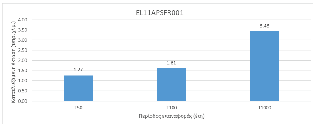
Σχήμα 3-5: Κατακλυζόμενες εκτάσεις ΖΔΥΚΠ EL11APSFR001 για τις πλημμύρες περιόδου επαναφοράς 50, 100 και 1.000 ετών
