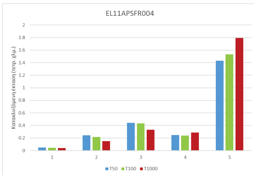
Σχήμα 3-23: Κατακλυζόμενη έκταση που αντιστοιχεί σε κάθε κατηγορία του δείκτη Επικινδυνότητας Πλημμύρας (κλάση Βαθμού Επιρροής Πλημμύρας), ανά εξεταζόμενο σενάριο στο σύνολο της ΖΔΥΚΠ EL11APSFR004
