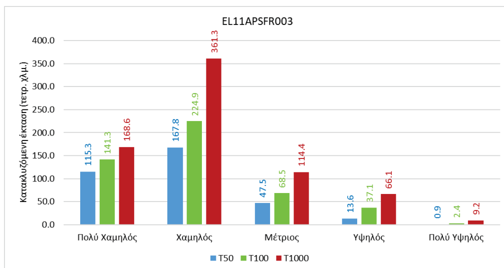
Σχήμα 3-21: Κατακλυζόμενη έκταση που αντιστοιχεί σε κάθε κατηγορία του δείκτη Κινδύνου Πλημμύρας (κλάση Μεγέθους Επιπτώσεων Πλημμύρας), ανά εξεταζόμενο σενάριο στη ΖΔΥΚΠ EL11APSR003
