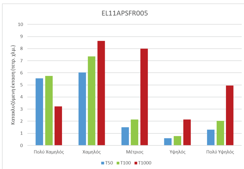
Σχήμα 3-26: Κατακλυζόμενη έκταση που αντιστοιχεί σε κάθε κατηγορία του δείκτη Επικινδυνότητας Πλημμύρας (κλάση Βαθμού Επιρροής Πλημμύρας), ανά εξεταζόμενο σενάριο στο σύνολο της ΖΔΥΚΠ EL11APSR005
