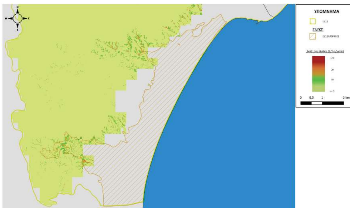
Εικόνα 3-31: Χάρτης εδαφικής απώλειας (SE) στην λεκάνη απορροής του ποταμού Στρυμόνα για την ΖΔΥΚΠ EL11APSF001
