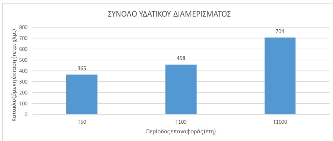
Σχήμα 3-4: Κατακλυζόμενες εκτάσεις ΥΔ για τις πλημμύρες περιόδου επαναφοράς 50, 100 και 1.000 ετών
