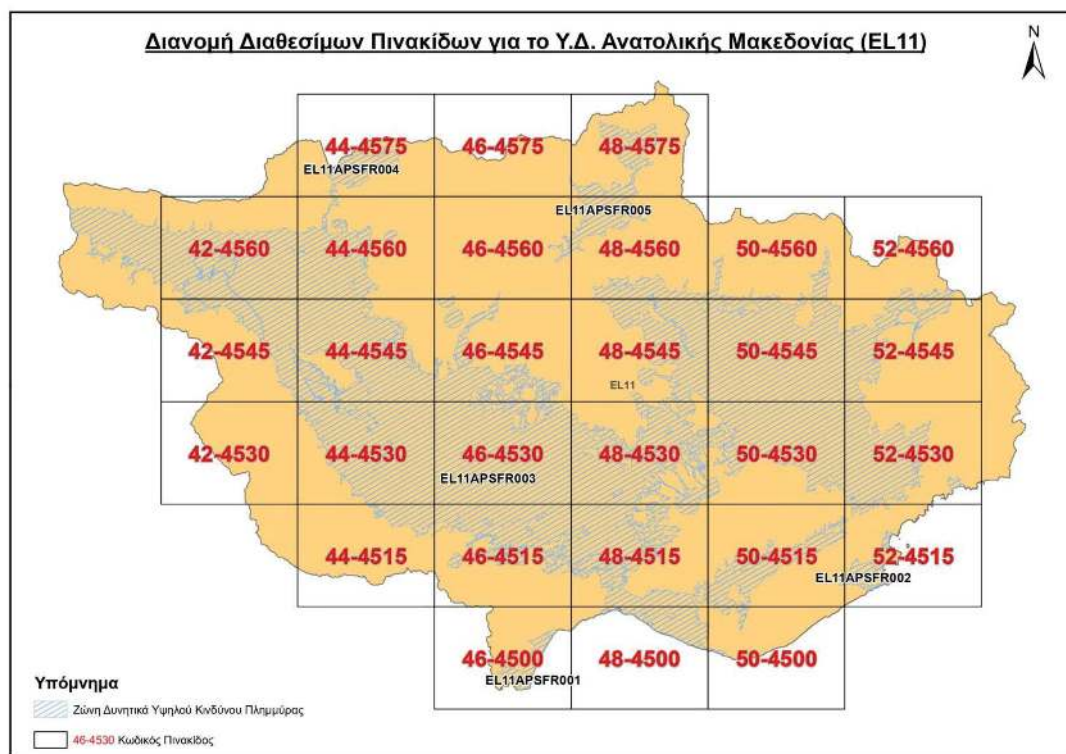
Εικόνα 3-24: Διανομή πινακίδων πλημμύρας από ποτάμια ροές
