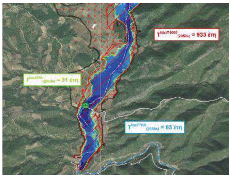
Εικόνα 3-54: Αντιστοίχιση της περιόδου επαναφοράς σε συνθήκες κλιματικής αλλαγής εντός των Χαρτών Επίδρασης Κλιματικής Αλλαγής, παράδειγμα εφαρμογής στο ΥΔ11
