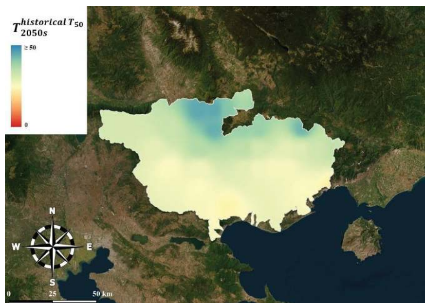
Εικόνα 3-48: Θεματικός χάρτης της χωρικής κατανομής των νέων περιόδων επαναφοράς T_{2050s}^{historical T_x} , για την κλιματική περίοδο 2041-01-01 έως 2070-12-31 (2050s), των γεγονότων βροχής που κατά την τρέχουσα περίοδο αντιστοιχούν σε περιόδους επαναφοράς T = 50 έτη.
