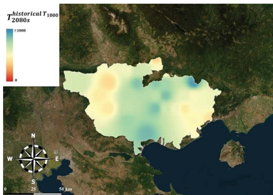
Εικόνα 3-53: Θεματικός χάρτης της χωρικής κατανομής των νέων περιόδων επαναφοράς T_{2080s}^{historicalTx} , για την κλιματική περίοδο 2071-01-01 έως 2100-12-31 (2080s), των γεγονότων βροχής που κατά την τρέχουσα περίοδο αντιστοιχούν σε περιόδους επαναφοράς T = 1000 έτη.
