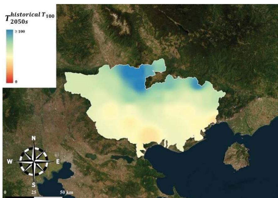
Εικόνα 3-49: Θεματικός χάρτης της χωρικής κατανομής των νέων περιόδων επαναφοράς T_{2050s}^{historical T_x} , για την κλιματική περίοδο 2041-01-01 έως 2070-12-31 (2050s), των γεγονότων βροχής που κατά την τρέχουσα περίοδο αντιστοιχούν σε περιόδους επαναφοράς T = 100 έτη.
