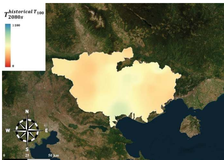
Εικόνα 3-52: Θεματικός χάρτης της χωρικής κατανομής των νέων περιόδων επαναφοράς T_{2080s}^{historicalTx} , για την κλιματική περίοδο 2071-01-01 έως 2100-12-31 (2080s), των γεγονότων βροχής που κατά την τρέχουσα περίοδο αντιστοιχούν σε περιόδους επαναφοράς T = 100 έτη.
