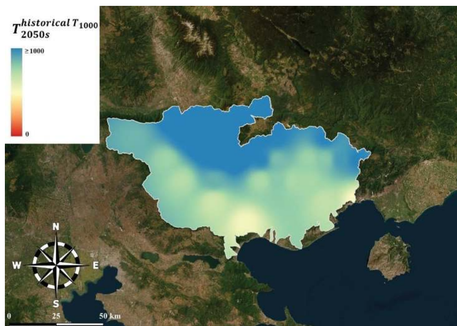
Εικόνα 3-50: Θεματικός χάρτης της χωρικής κατανομής των νέων περιόδων επαναφοράς T_{2050s}^{historical T_x} , για την κλιματική περίοδο 2041-01-01 έως 2070-12-31 (2050s), των γεγονότων βροχής που κατά την τρέχουσα περίοδο αντιστοιχούν σε περιόδους επαναφοράς T = 1000 έτη.
