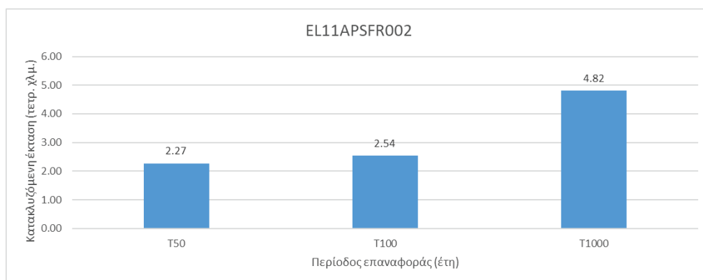
Σχήμα 3-6: Κατακλυζόμενες εκτάσεις ΖΔΥΚΠ EL11APSFR002 για τις πλημμύρες περιόδου επαναφοράς 50, 100 και 1.000 ετών
