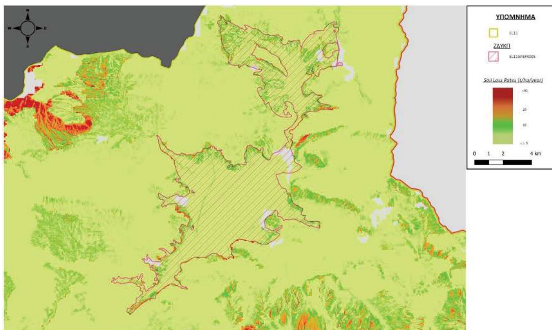
Εικόνα 3-35: Χάρτης εδαφικής απώλειας (SE) στην λεκάνη απορροής του ποταμού Στρυμόνα για την ΖΔΥΚΠ EL11APSF005
