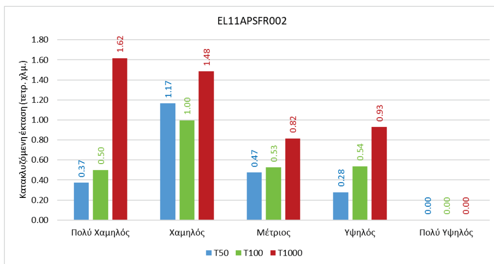
Σχήμα 3-17: Κατακλυζόμενη έκταση που αντιστοιχεί σε κάθε κατηγορία του δείκτη Επικινδυνότητας Πλημμύρας (κλάση Βαθμού Επιρροής Πλημμύρας), ανά εξεταζόμενο σενάριο στο σύνολο της ΖΔΥΚΠ EL11APSFR002
