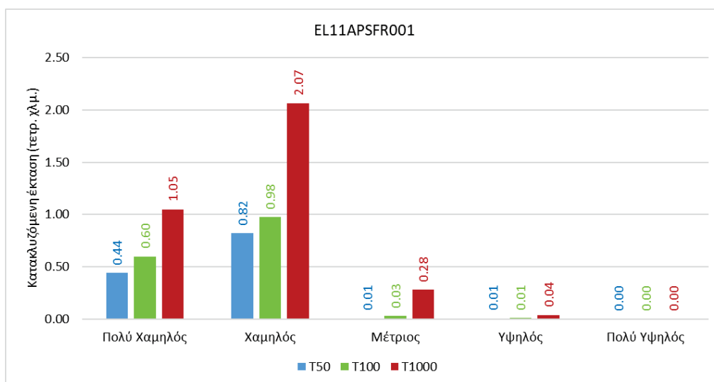
Εικόνα 4-1: Έκταση που αντιστοιχεί σε κάθε κατηγορία κινδύνου πλημμύρας, ανά περίοδο επαναφοράς (ΖΔΥΚΠ EL11APSFR001)
