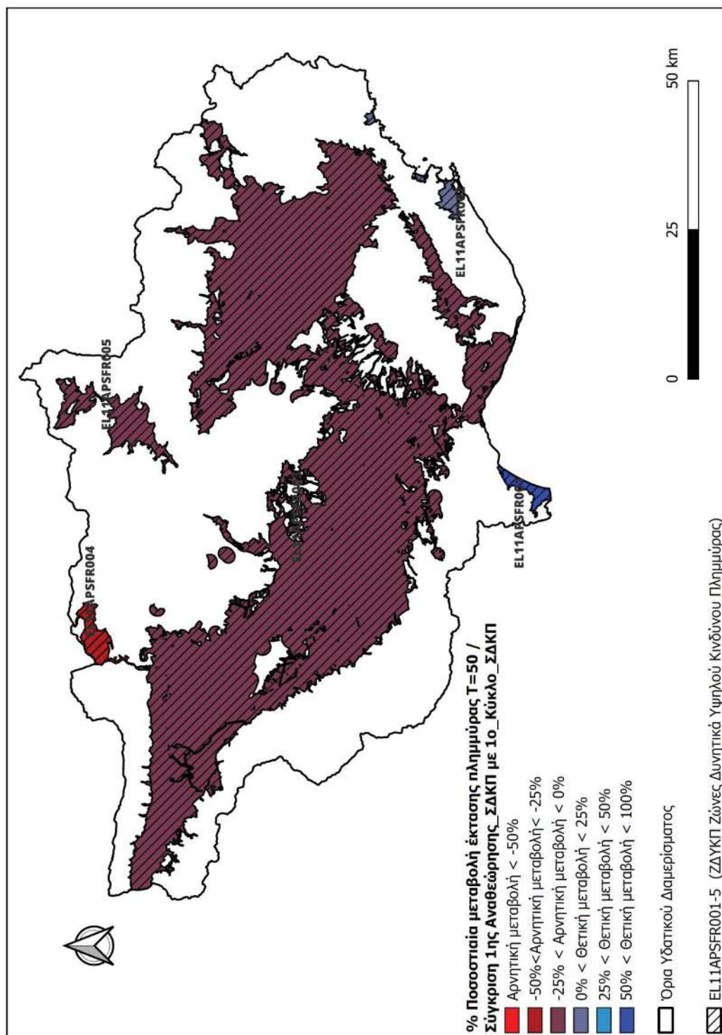
Εικόνα 3-62: Σύγκριση εκτάσεων πλημμύρας (%μεταβολή) (1ος κύκλος/ 1η Αναθ.) σε επίπεδο ΖΔΥΚΠ για T=50 έτη
