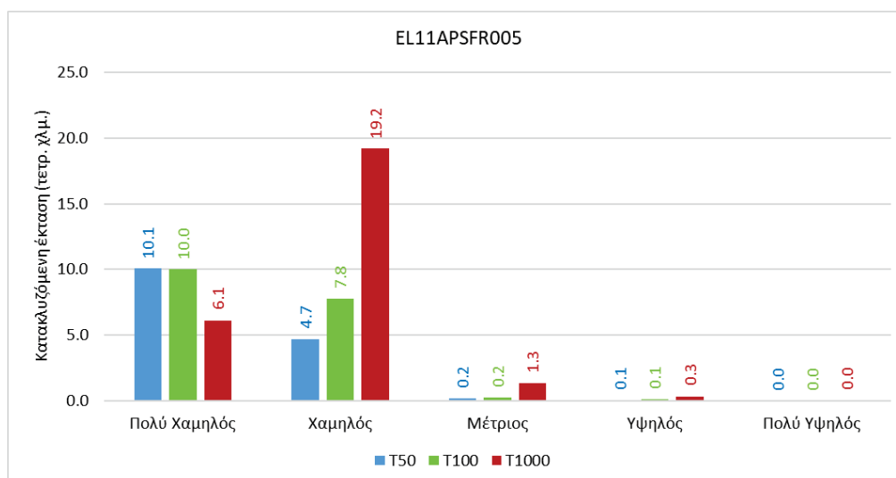
Σχήμα 3-27: Κατακλυζόμενη έκταση που αντιστοιχεί σε κάθε κατηγορία του δείκτη Κινδύνου Πλημμύρας (κλάση Μεγέθους Επιπτώσεων Πλημμύρας), ανά εξεταζόμενο σενάριο στη ΖΔΥΚΠ EL11APSF005
