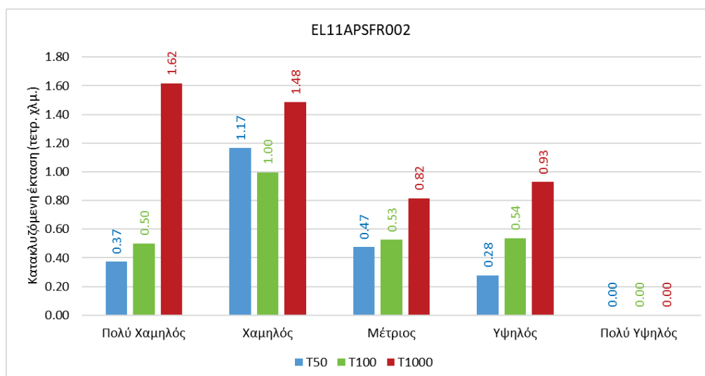
Σχήμα 3-18: Κατακλυζόμενη έκταση που αντιστοιχεί σε κάθε κατηγορία του δείκτη Κινδύνου Πλημμύρας (κλάση Μεγέθους Επιπτώσεων Πλημμύρας), ανά εξεταζόμενο σενάριο στη ΖΔΥΚΠ EL11APSF002
