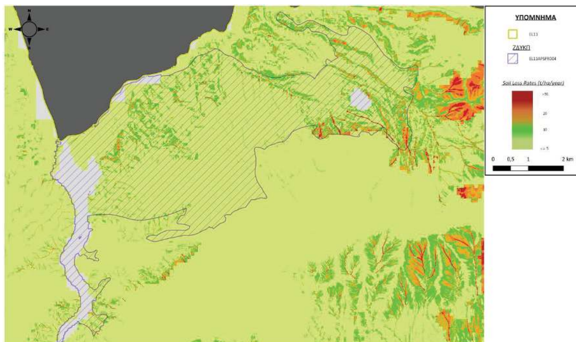
Εικόνα 3-34: Χάρτης εδαφικής απώλειας (SE) στην λεκάνη απορροής του ποταμού Στρυμόνα για την ΖΔΥΚΠ EL11APSFR004
