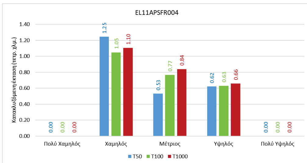
Εικόνα 4-4: Έκταση που αντιστοιχεί σε κάθε κατηγορία κινδύνου πλημμύρας, ανά περίοδο επαναφοράς (ΖΔΥΚΠ EL11APSFR004)
