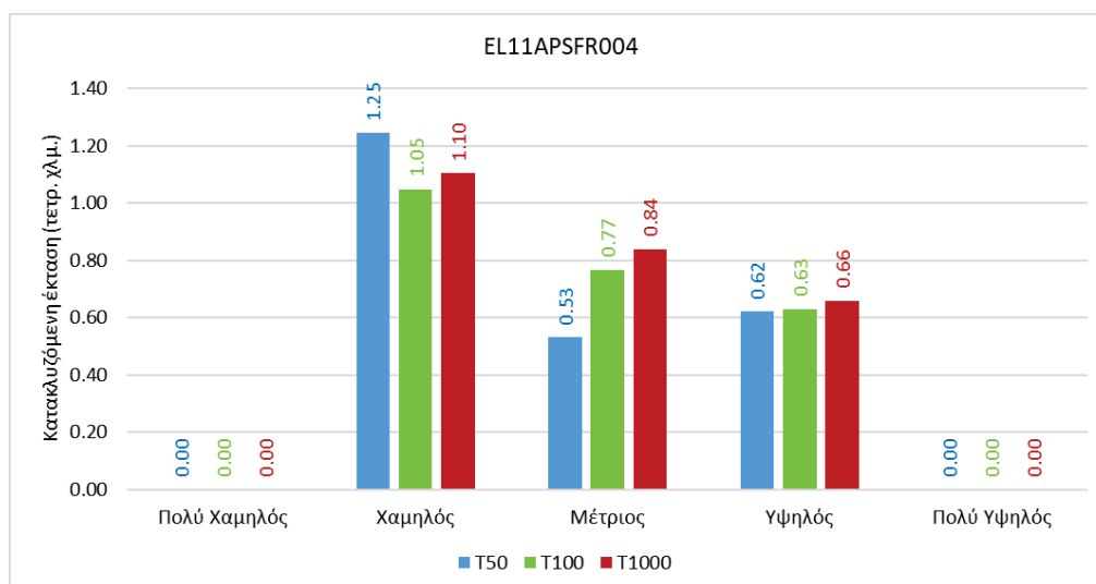
Σχήμα 3-24: Κατακλυζόμενη έκταση που αντιστοιχεί σε κάθε κατηγορία του δείκτη Κινδύνου Πλημμύρας (κλάση Μεγέθους Επιπτώσεων Πλημμύρας), ανά εξεταζόμενο σενάριο στη ΖΔΥΚΠ EL11APSFR004
