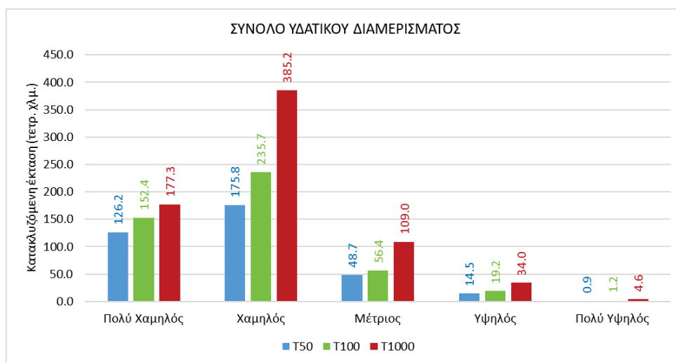
Σχήμα 3-12: Κατακλυζόμενη έκταση που αντιστοιχεί σε κάθε κατηγορία του δείκτη Κινδύνου Πλημμύρας (κλάση Μεγέθους Επιπτώσεων Πλημμύρας), ανά εξεταζόμενο σενάριο στο σύνολο του ΥΔ11
