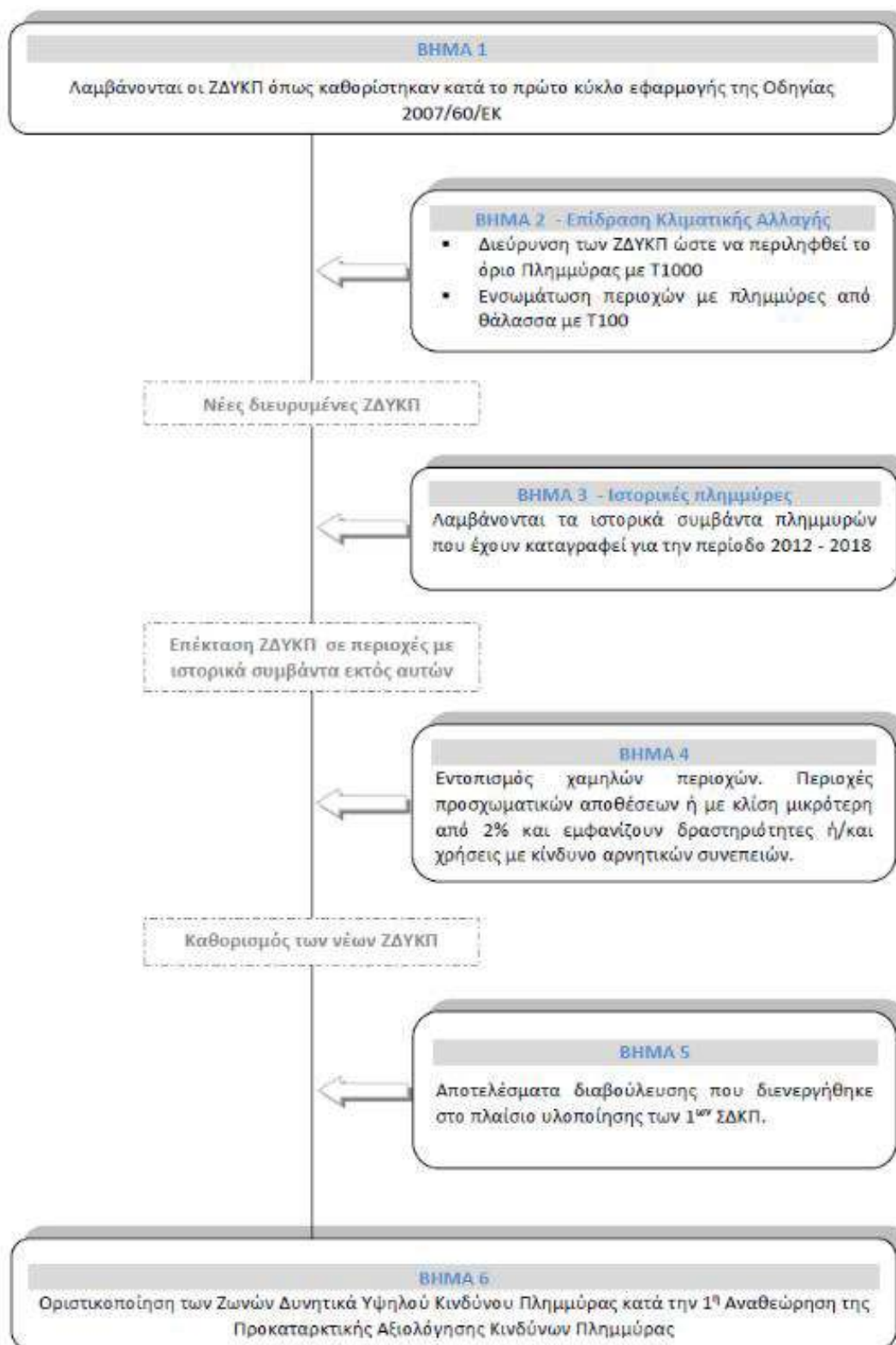
Σχήμα 3-3: Σχηματοποιημένη παρουσίαση της προσέγγισης αναθεώρησης των ΖΔΥΚΠ
