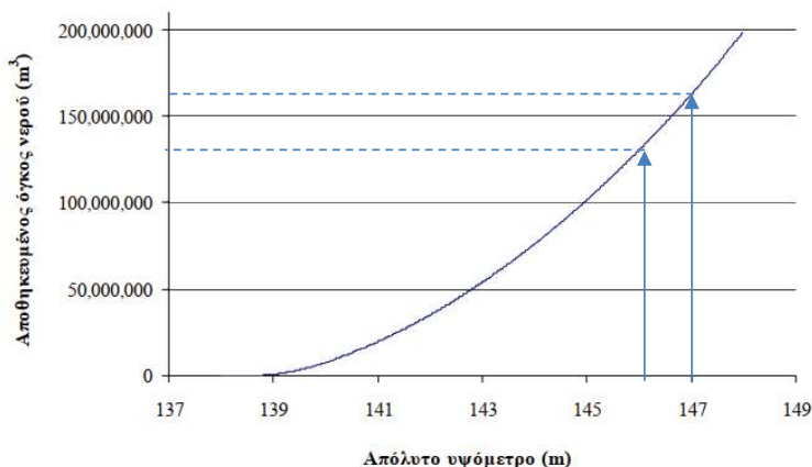
Εικόνα 3-35: Διάγραμμα στάθμης-όγκου λίμνης Δοϊράνης (Αξιολόγηση των υδροτοπικών λειτουργιών και αξιών της διασυνοριακής Λίμνης Δοϊράνης, ΕΚΒΥ 2004). Ενδείξεις όγκου σε χαρακτηριστικές στάθμες.
