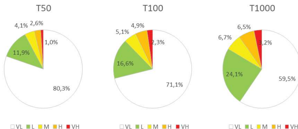
Εικόνα 3-43: Εκτάσεις ανά κατηγορία κινδύνου πλημμύρας στη ΖΔΥΚΠ EL10APSF008 για T50, T100 και T1000
