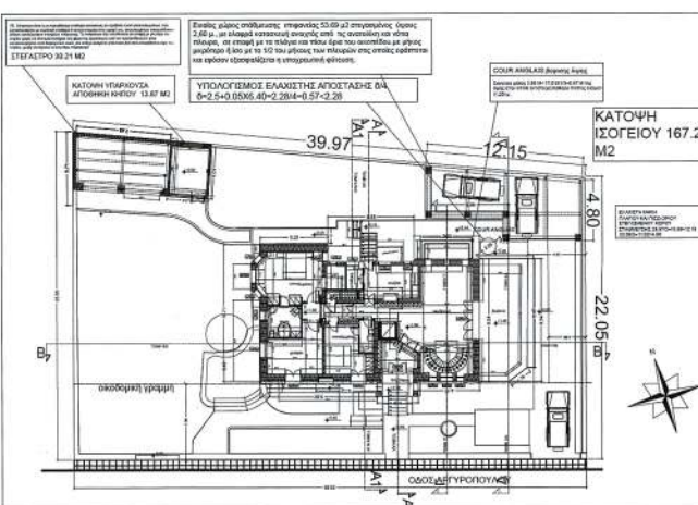
ΣΧΕΔΙΟ 3 ΚΑΤΟΨΗ ΙΣΟΓΕΙΟΥ
