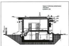
ΤΟΜΗ ΓΓ
