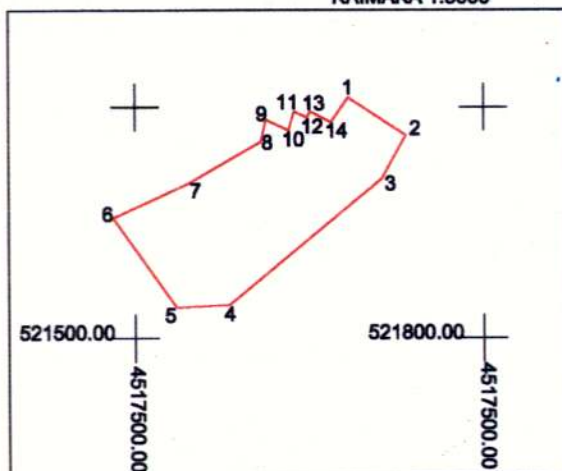
ΤΟΠΟΓΡΑΦΙΚΟ ΔΙΑΓΡΑΜΜΑ ΚΛΙΜΑΚΑ 1:5000
