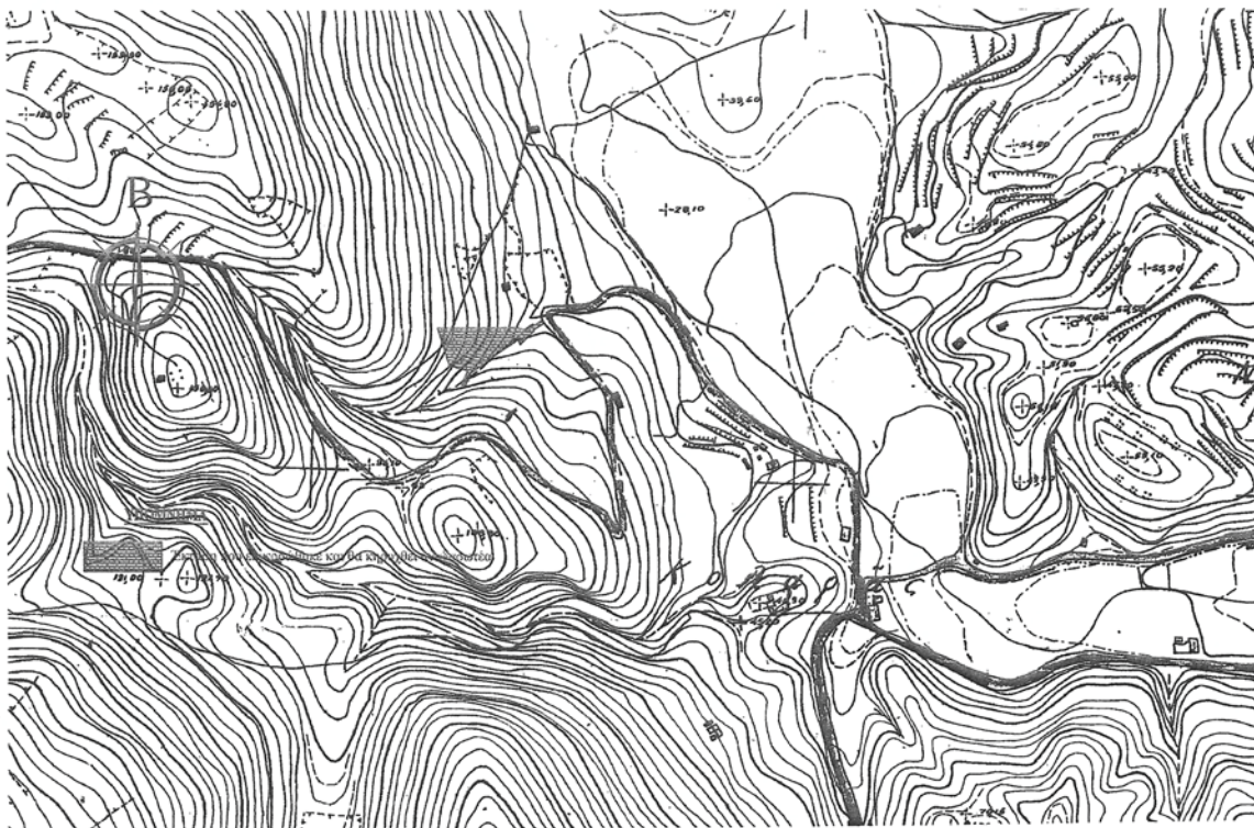
ΤΟΠΟΓΡΑΦΙΚΟ ΔΙΑΓΡΑΜΜΑ ΚΛΙΜΑΚΑΣ 1:1.250 ΤΗΣ ΕΚΤΑΣΗΣ ΠΟΥ ΕΚΧΕΡΣΩΘΗΚΕ ΣΤΗ ΘΕΣΗ ΜΑΡΑΘΕΑ ΤΗΣ ΤΟΠΙΚΗΣ ΚΟΙΝΟΤΗΤΑΣ ΜΑΡΑΘΕΑΣ ΤΟΥ ΔΗΜΟΥ ΑΝΑΤΟΛΙΚΗΣ ΜΑΝΗΣ.
