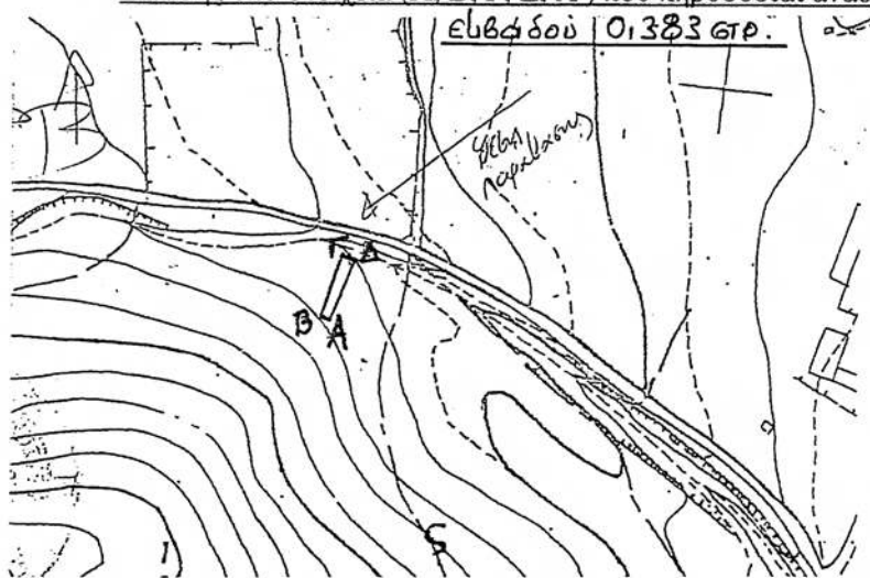
Τοπογραφικό διάγραμμα της έκτασης σε κλιμ. 1:500 με τα ίδια στοιχεία
