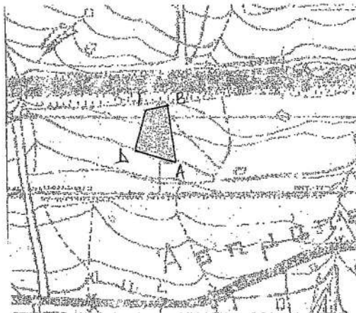
Τοπογραφικό Διάγραμμα της έκτασης κλιμ. 1:1000
