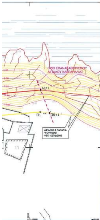
ΑΠΟΣΠΑΣΜΑ ΤΟΠΟΓΡΑΦΙΚΟΥ ΔΙΑΓΡΑΜΜΑΤΟΣ Γ.Υ.Σ. "ΕΜΠΛΥΣΗ" Δ. & ΦΙΣΚΑΡΟΥ ΔΗΜΟΥ ΕΡΙΣΟΥ ΝΟΜΟΥ ΚΕΦΑΛΛΗΝΙΑΣ ΑΡ. Π.Π.123 - ΚΑΙΜΑΚΑ 1:50.000 (ΘΑΚΗ)
