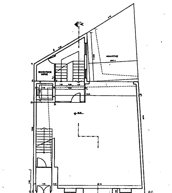
ΚΑΤΩΦΗ ΙΣΟΓΕΙΟΥ PARKING ΟΔΟΣ ΚΟΡΥΖΗ
