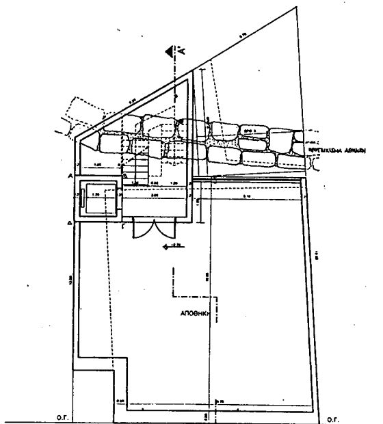
ΚΑΤΩΦΗ ΥΠΟΓΕΙΟΥ ΟΔΟΣ ΚΟΡΥΖΗ
