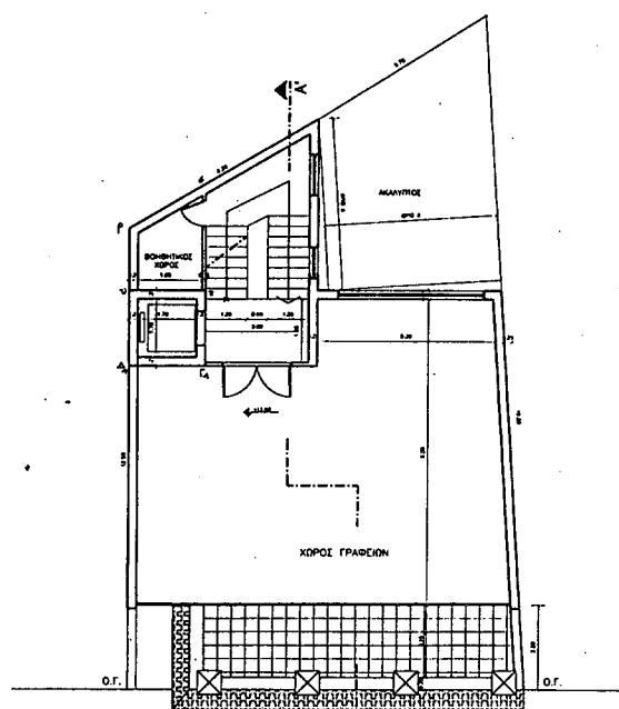
ΚΑΤΩΦΗ Δ' ΟΡΟΦΟΥ ΟΔΟΣ ΚΟΡΥΖΗ
