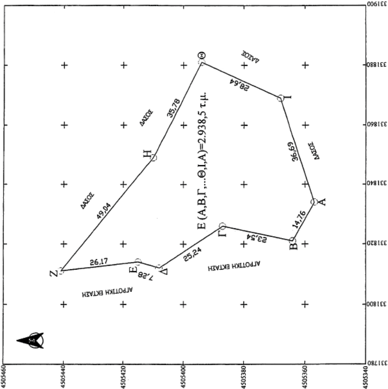
ΤΟΠΟΓΡΑΦΙΚΟ ΔΙΑΓΡΑΜΜΑ ΕΚΧΕΡΣΩΘΕΙΣΑΣ ΕΚΤΑΣΗΣ ΣΤΗ ΘΕΣΗ "ΝΤΑΜΦΟΡ", ΛΙΩΤΙΚΟΥ ΔΑΣΟΥΣ Μ. ΡΕΜΑΤΟΣ, ΔΗΜΟΥ ΝΑΟΥΣΑΣ ΚΛΙΜΑΚΑ 1:1.000
