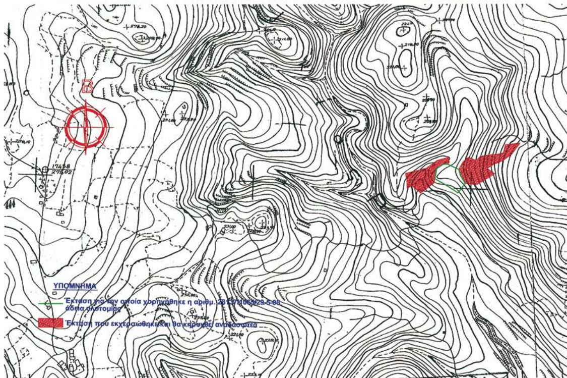
ΤΟΠΟΓΡΑΦΙΚΟ ΔΙΑΓΡΑΜΜΑ ΚΛΙΜΑΚΑΣ 1:1.250 ΤΗΣ ΕΚΤΑΣΗΣ ΠΟΥ ΕΚΧΕΡΣΩΘΗΚΕ ΣΤΗ ΘΕΣΗ ΟΡΓΗ Η' ΟΡΓΙΕΣ ΤΟΥ Δ.Δ. ΜΥΡΙΝΗΣ ΠΕΡΙΦΕΡΕΙΑΣ ΔΗΜΟΥ ΓΥΘΕΙΟΥ.
