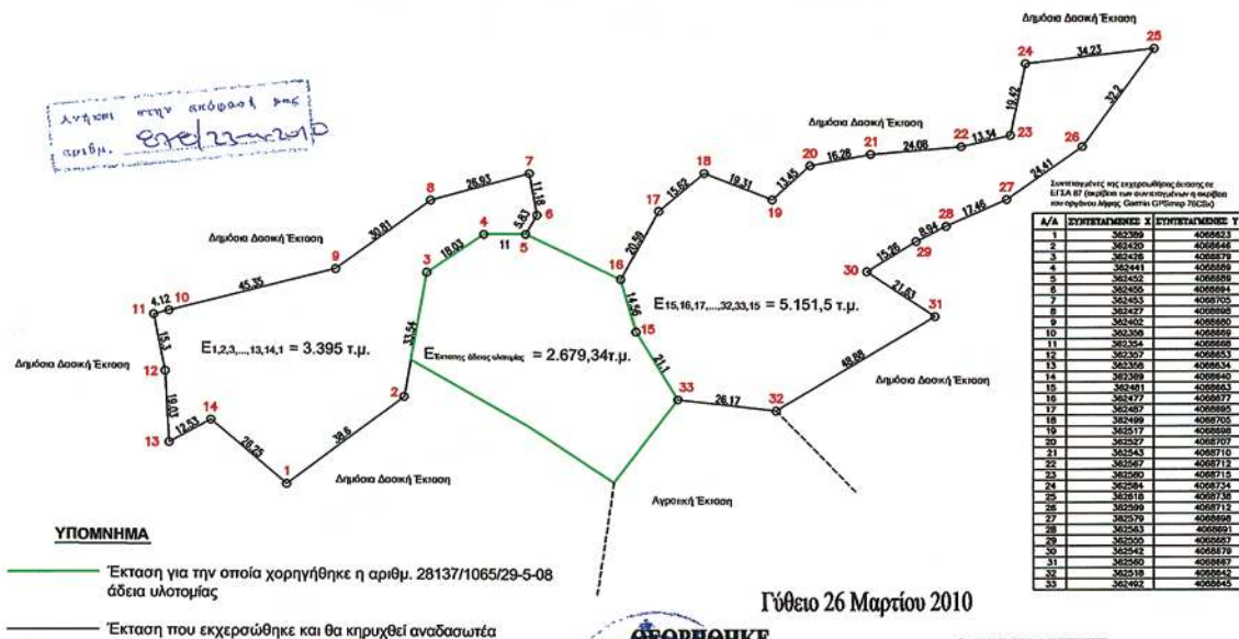
ΤΟΠΟΓΡΑΦΙΚΟ ΔΙΑΓΡΑΜΜΑ ΚΛΙΜΑΚΑΣ 1:1.250 ΤΗΣ ΕΚΤΑΣΗΣ ΠΟΥ ΕΚΧΕΡΣΩΘΗΚΕ ΣΤΗ ΘΕΣΗ ΟΡΓΗ Η' ΟΡΓΙΕΣ ΤΟΥ Δ.Δ. ΜΥΡΙΝΗΣ ΠΕΡΙΦΕΡΕΙΑΣ ΔΗΜΟΥ ΓΥΘΕΙΟΥ.
