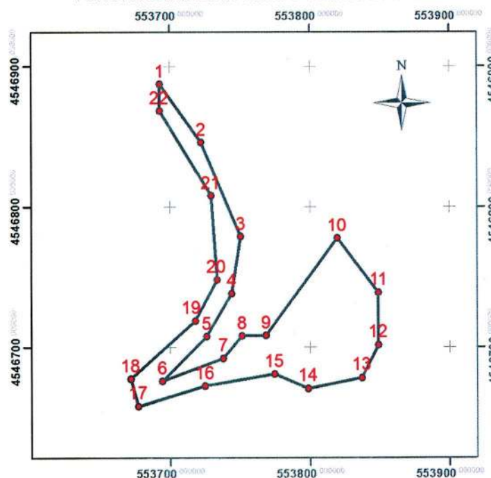
ΤΟΠΟΓΡΑΦΙΚΟ ΔΙΑΓΡΑΜΜΑ - ΚΛΙΜΑΚΑ 1:3.000
