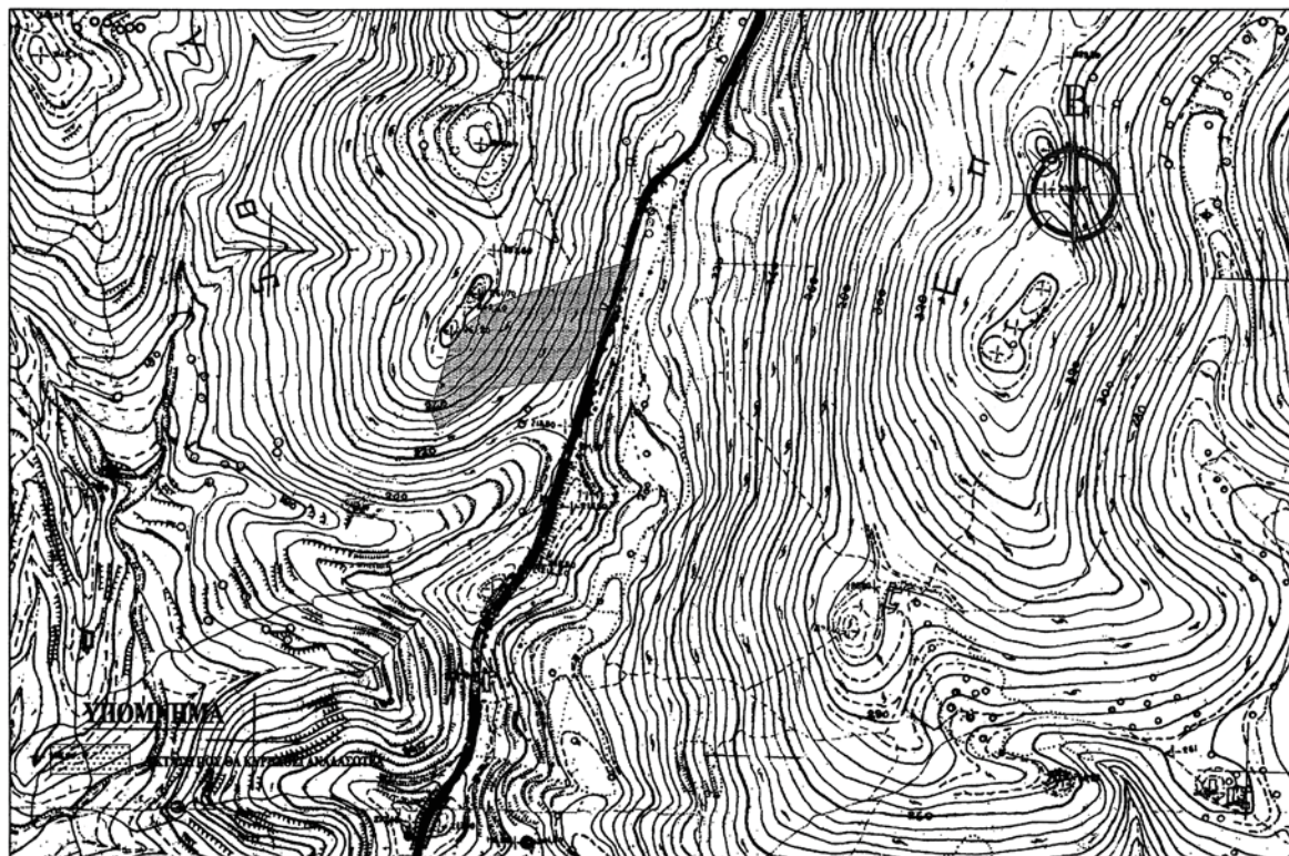
ΤΟΠΟΓΡΑΦΙΚΟ ΔΙΑΓΡΑΜΜΑ ΚΛΙΜΑΚΑΣ 1:2.500 ΤΗΣ ΕΚΤΑΣΗΣ ΠΟΥ ΚΑΗΚΕ ΣΤΙΣ 10-8-2010 ΣΤΗ ΘΕΣΗ ΣΩΡΟΣ ΤΟΥ Δ.Δ. ΠΕΤΡΙΝΑΣ ΠΕΡΙΦΕΡΕΙΑΣ ΔΗΜΟΥ ΣΜΥΝΟΥΣ.
