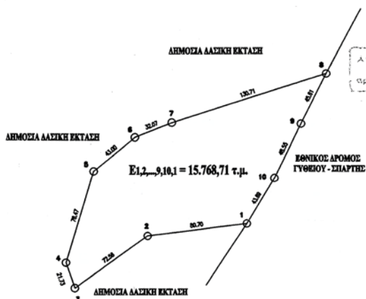
ΤΟΠΟΓΡΑΦΙΚΟ ΔΙΑΓΡΑΜΜΑ ΚΛΙΜΑΚΑΣ 1:2.500 ΤΗΣ ΕΚΤΑΣΗΣ ΠΟΥ ΚΑΗΚΕ ΣΤΙΣ 10-8-2010 ΣΤΗ ΘΕΣΗ ΣΩΡΟΣ ΤΟΥ Δ.Δ. ΠΕΤΡΙΝΑΣ ΠΕΡΙΦΕΡΕΙΑΣ ΔΗΜΟΥ ΣΜΥΝΟΥΣ.
