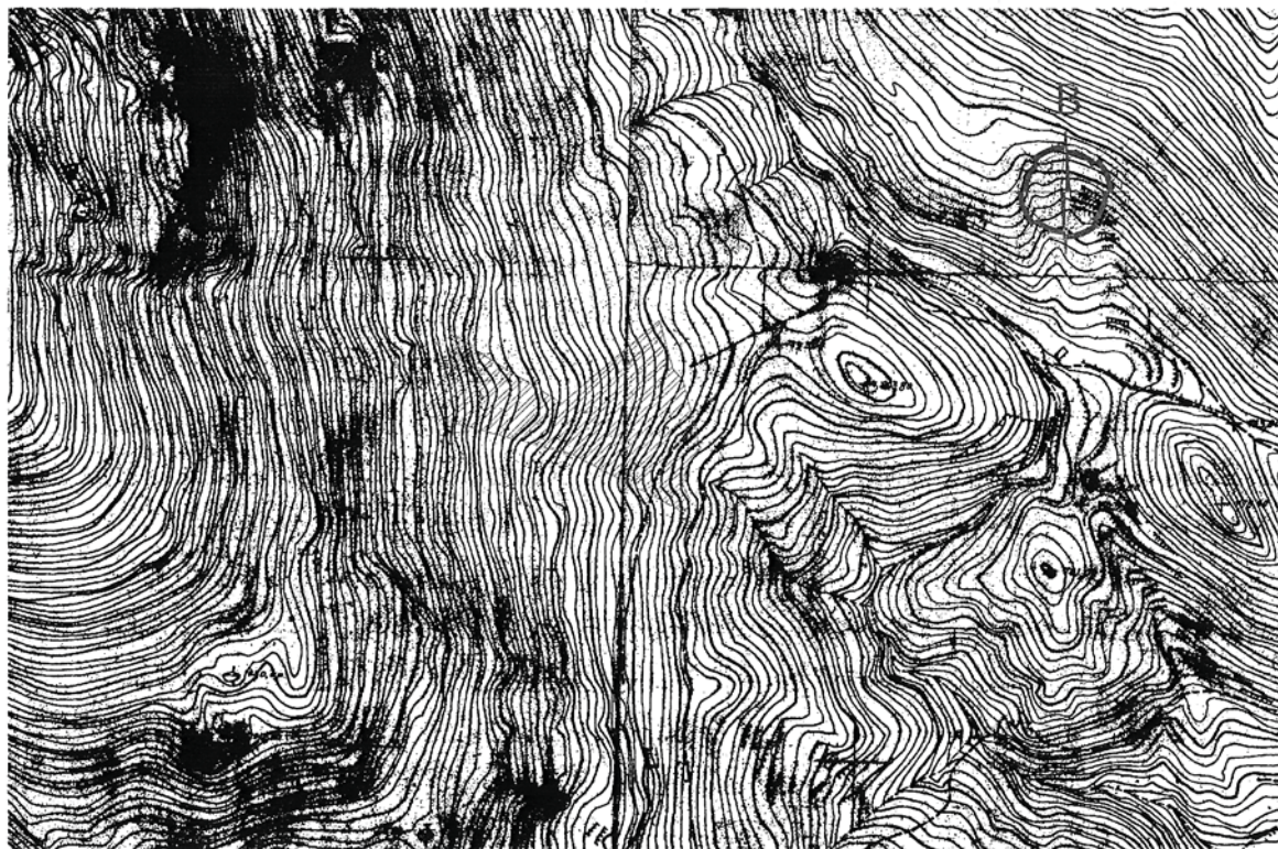
ΤΟΠΟΓΡΑΦΙΚΟ ΔΙΑΓΡΑΜΜΑ ΚΛΙΜΑΚΑΣ 1:2.500 ΤΗΣ ΕΚΤΑΣΗΣ ΠΟΥ ΚΑΗΚΕ ΣΤΙΣ 2-12-2010 ΣΤΗ ΘΕΣΗ ΣΠΑΝΗ ΡΑΧΗ ΤΟΥ Δ.Δ. ΣΙΔΗΡΟΚΑΣΤΡΟΥ ΠΕΡΙΦΕΡΕΙΑΣ ΔΗΜΟΥ ΓΥΘΕΙΟΥ.
