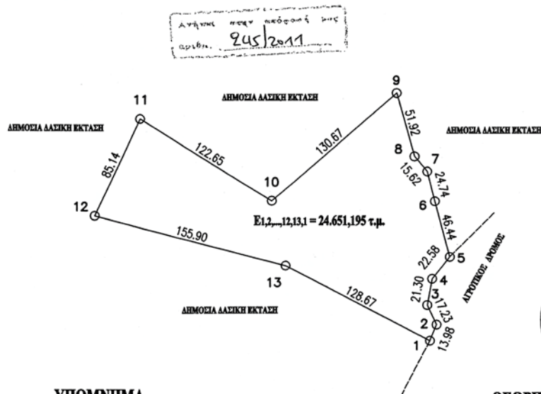
ΤΟΠΟΓΡΑΦΙΚΟ ΔΙΑΓΡΑΜΜΑ ΚΛΙΜΑΚΑΣ 1:2.500 ΤΗΣ ΕΚΤΑΣΗΣ ΠΟΥ ΚΑΗΚΕ ΣΤΙΣ 2-12-2010 ΣΤΗ ΘΕΣΗ ΣΠΑΝΗ ΡΑΧΗ ΤΟΥ Δ.Δ. ΣΙΔΗΡΟΚΑΣΤΡΟΥ ΠΕΡΙΦΕΡΕΙΑΣ ΔΗΜΟΥ ΓΥΘΕΙΟΥ.
