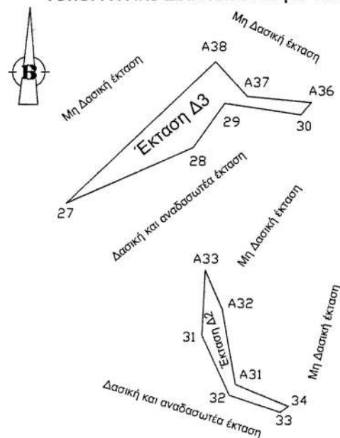
ΤΟΠΟΓΡΑΦΙΚΟ ΔΙΑΓΡΑΜΜΑ κλίμ.: 1:1000
