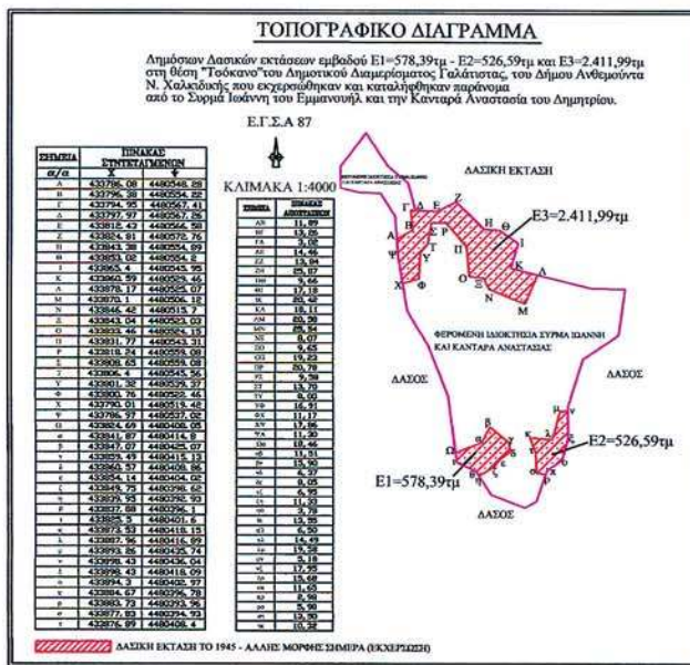
ΚΛΙΜΑΚΑ 1:4000
