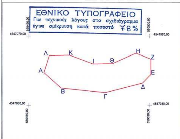
ΤΟΠΟΓΡΑΦΙΚΟ ΔΙΑΓΡΑΜΜΑ ΚΛΙΜΑΚΑ 1: 1.000
