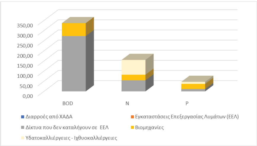
Σχήμα 5-7: Συνολικά ετήσια φορτία BOD, N και P που απορρέουν στη Λεκάνη Απορροής ΒΑ Παραλίας Καλλιδρόμου (EL0722) από σημειακές πηγές ρύπανσης
