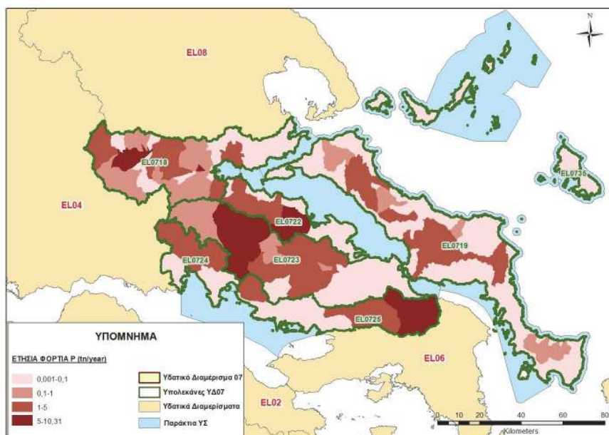
Χάρτης 5-47: Ετήσια επιφανειακά φορτία P που απορρέουν από όλες τις πηγές ρύπανσης στο ΥΔ Ανατολικής Στερέας Ελλάδας (EL07)
