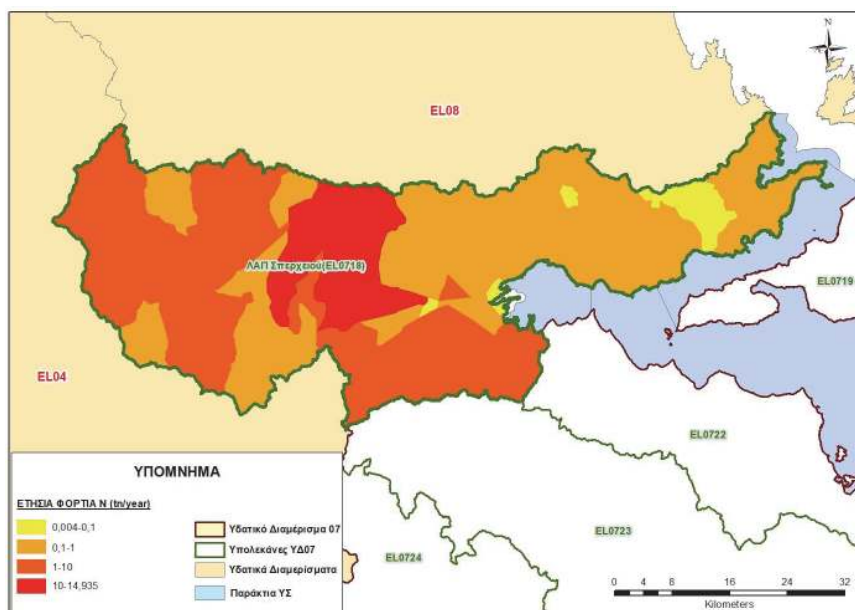
Χάρτης 5-28: Ετήσια φορτία Ν (t/year) που παράγονται στη Λεκάνη Απορροής Σπερχειού (EL0718) από διάχυτες πηγές ρύπανσης
