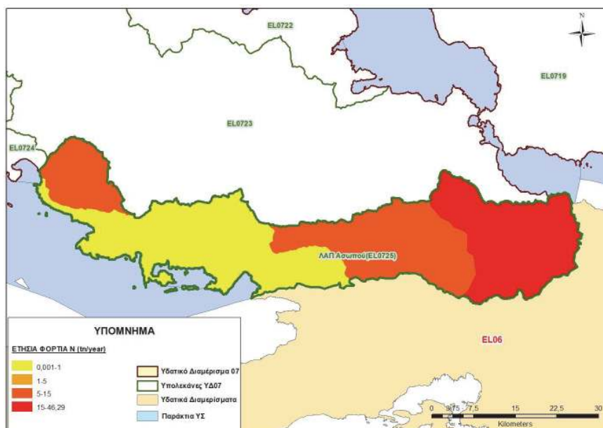
Χάρτης 5-64: Ετήσια επιφανειακά φορτία Ν που απορρέουν από όλες τις πηγές ρύπανσης στη Λεκάνη Απορροής Ασωπού (EL725)
