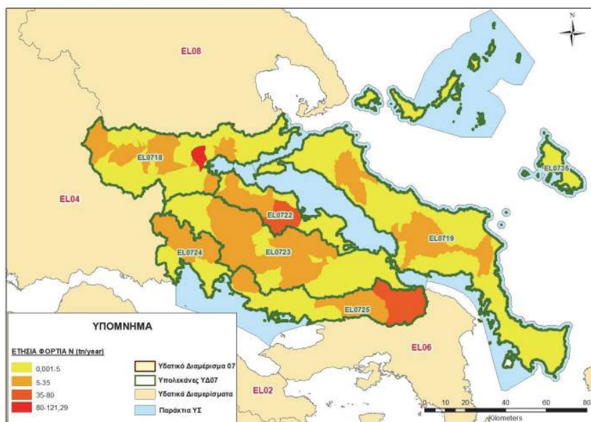
Χάρτης 5-46: Ετήσια επιφανειακά φορτία N που απορρέουν από όλες τις πηγές ρύπανσης στο ΥΔ Ανατολικής Στερέας Ελλάδας (EL07)
