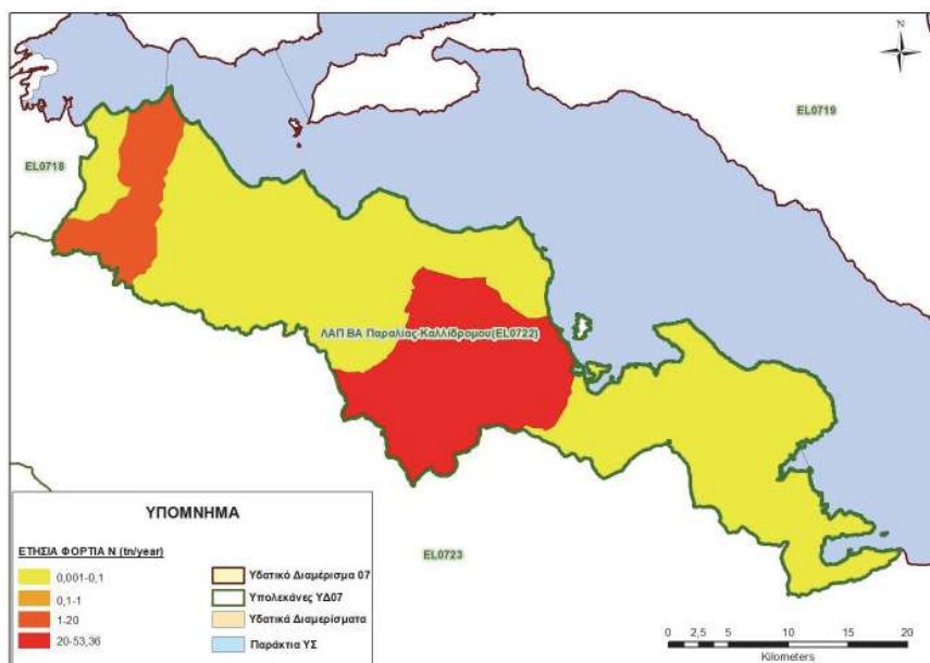
Χάρτης 5-12: Ετήσια φορτία Ν (tn/year) που παράγονται στη Λεκάνη Απορροής ΒΑ Παραλίας Καλλίδρομου (EL0722) από σημειακές πηγές ρύπανσης
