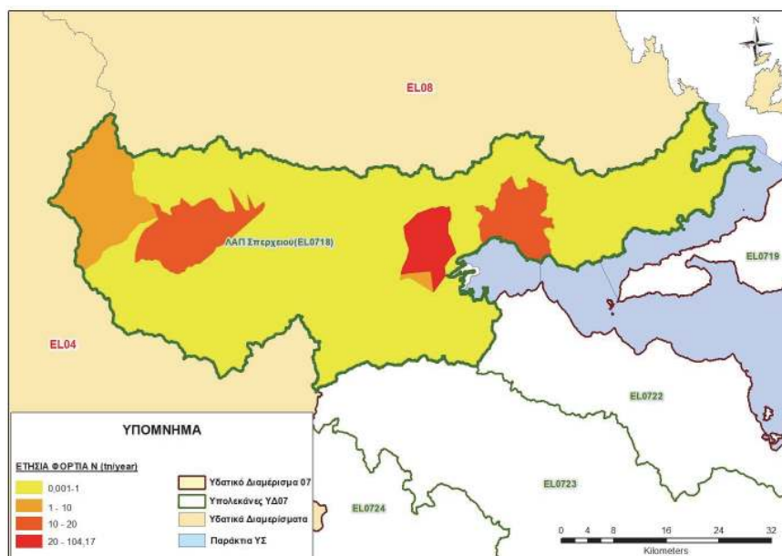
Χάρτης 5-6: Ετήσια φορτία N (tn/year) που παράγονται στη Λεκάνη Απορροής Σπερχείου (EL0718) από σημειακές πηγές ρύπανσης
