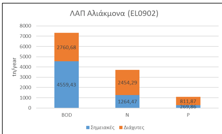
Διάγραμμα 5-15: Συνολικά ετήσια φορτία BOD, N και P που καταλήγουν σε ΥΣ της ΛΑΠ Αλιάκμονα (EL0902) από όλες τις πηγές ρύπανσης
